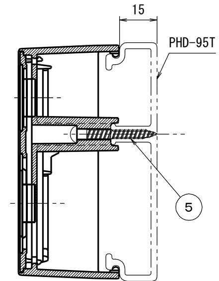
A-A断面図
